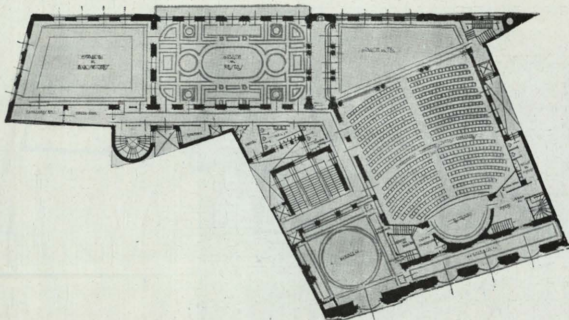
PLANTA PRINCIPAL.
